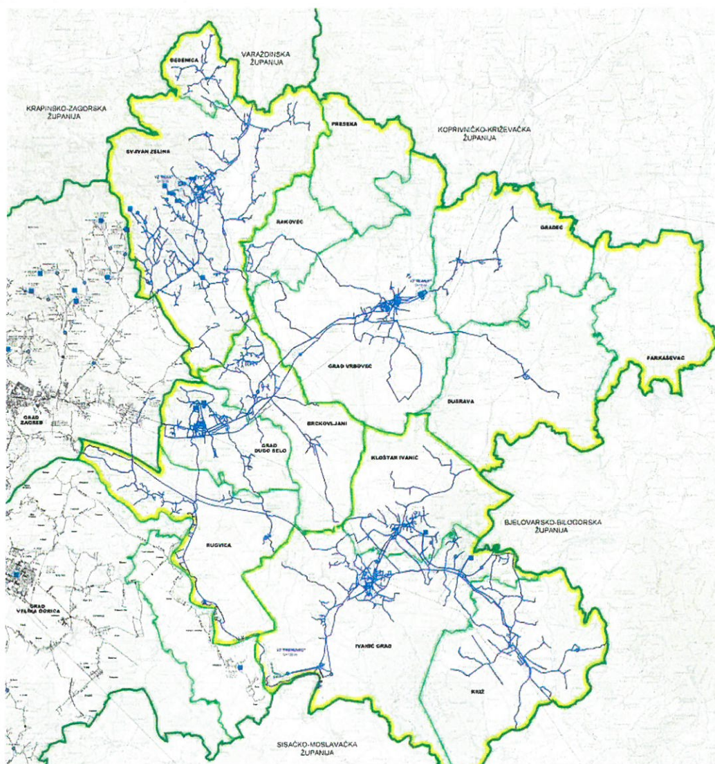
Prikaz postojeće konfiguracije vodoopskrbnog sustava VIOŽ
